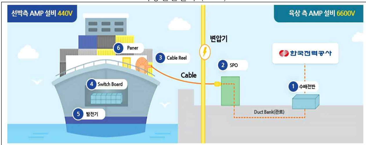
< 육상전원설비 (AMP) >
